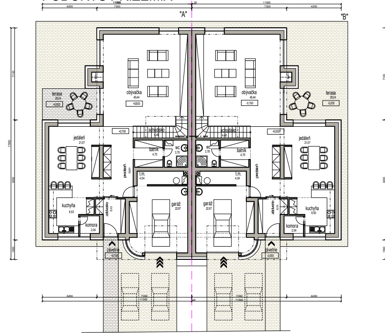
PODORYS PRÍZEMIA
