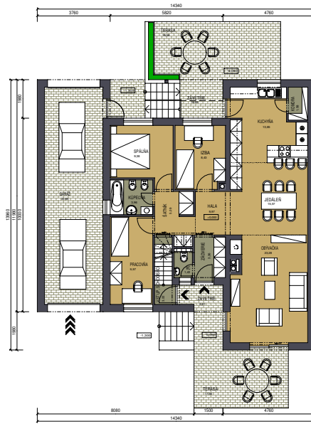
PODORYS PRÍZEMIA
