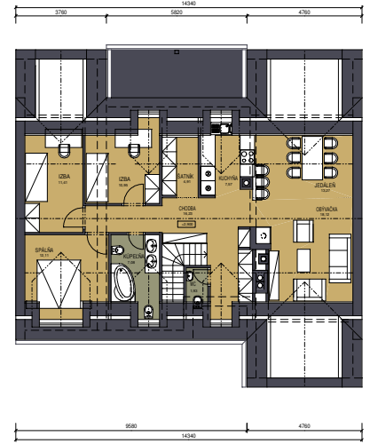
PODORYS PODKROVIA
