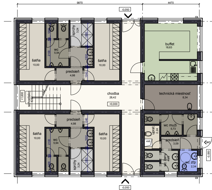
PODORYS PRÍZEMIA
