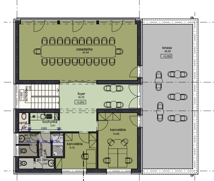
PODORYS POSCHODIA
